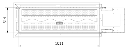
B-B ( 1 : 10 )
