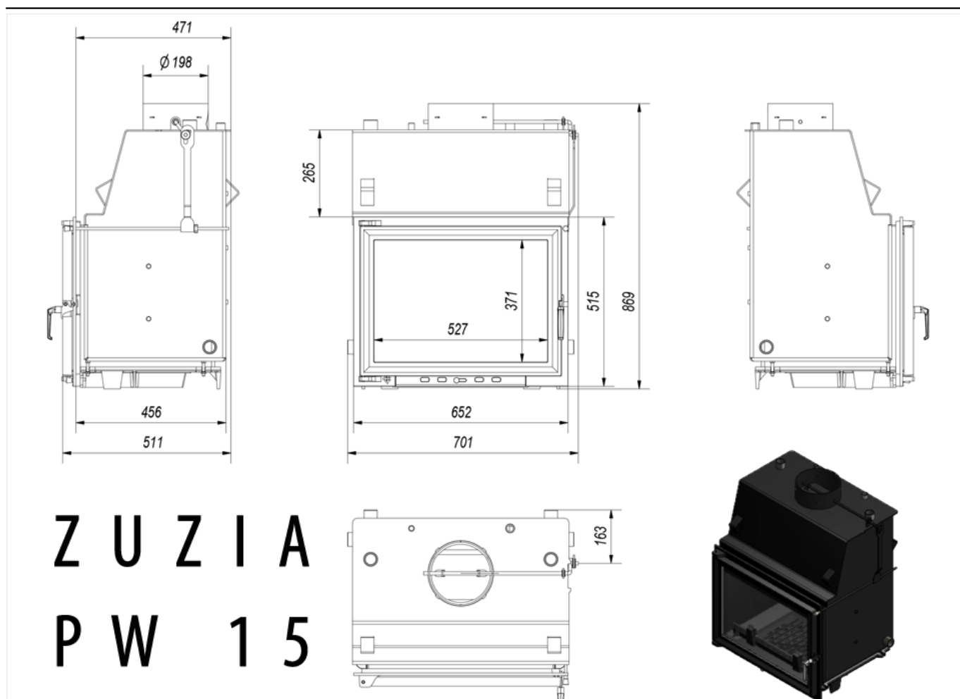
Wymiary wkładu 19kW
